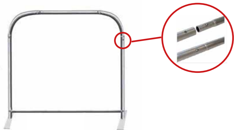
Innesto rapido. Tapered snap couplings.
